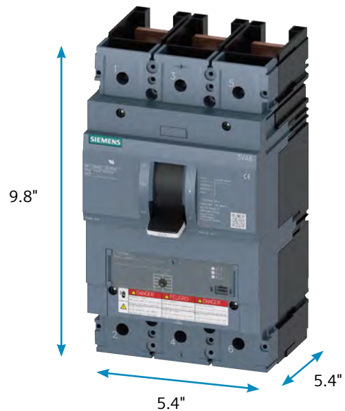
3VA64
